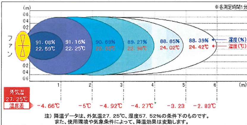
ミスト噴霧による周辺温度の降温目安 (WM-560[50Hz時]の冷風到達範囲)
